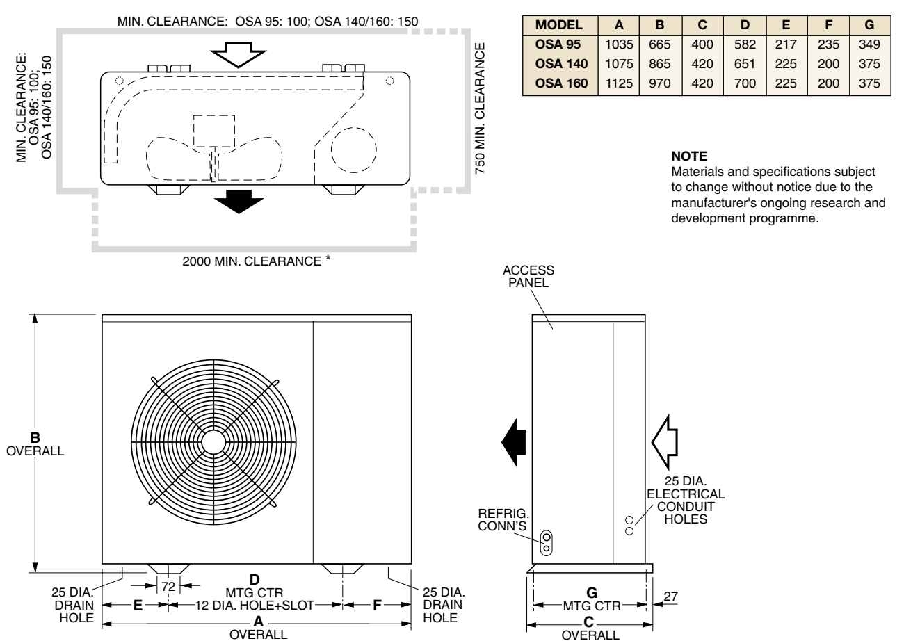
Fig. 2 OSA 95, 140, 160
